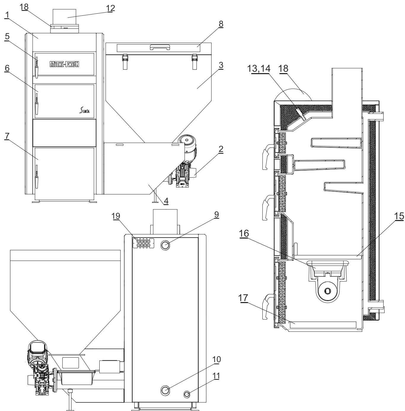
Рисунок 7.1 Основные элементы конструкции котла SMART, SMART EKO, SMART BIO
