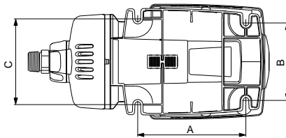
Рис. 5 Плита-основание
