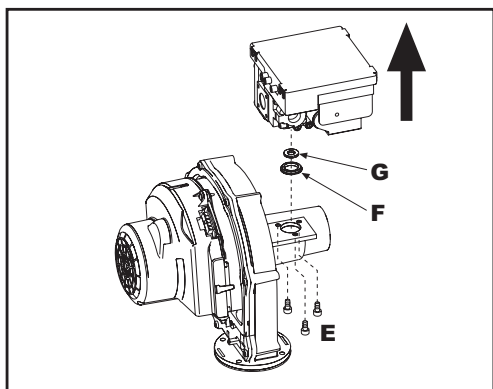
рис. 33 - Модель ENERGY TOP W 70 - W 80
