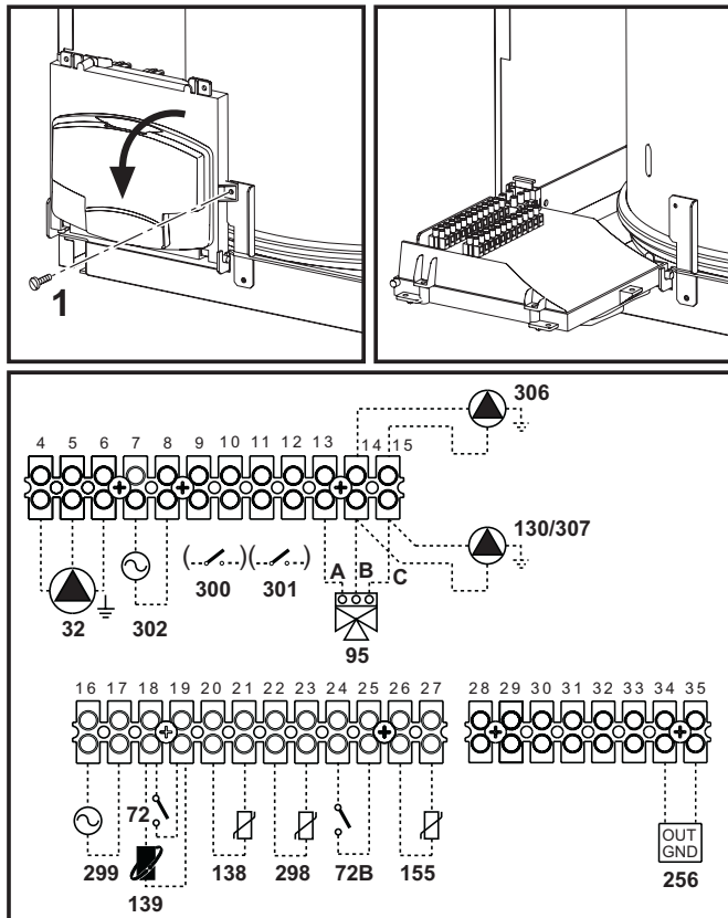
рис. 24 - Блок зажимов
