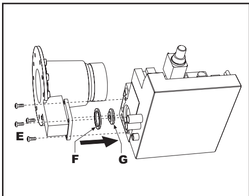
рис. 34 - Модель ENERGY TOP W 125
