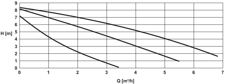
рис. 16 - Напор насоса
