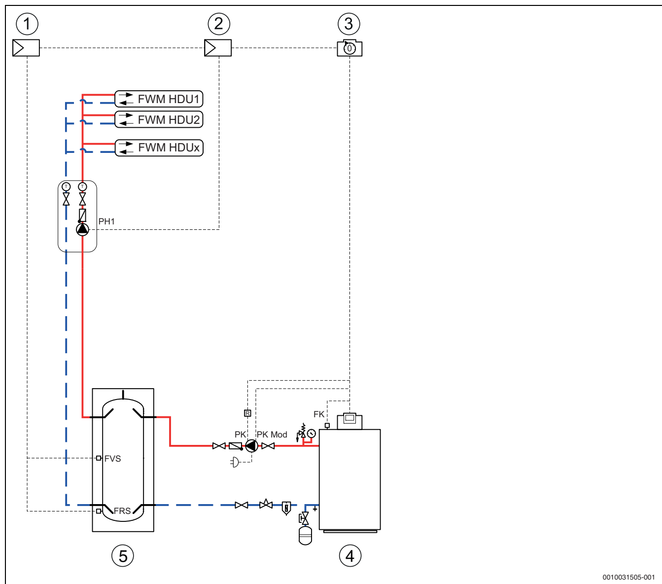
Рис. 28 Теплогенератор с горелкой, совместимой с котлом
