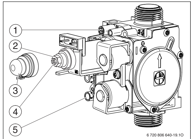
Рис. 31 Газовая арматура
