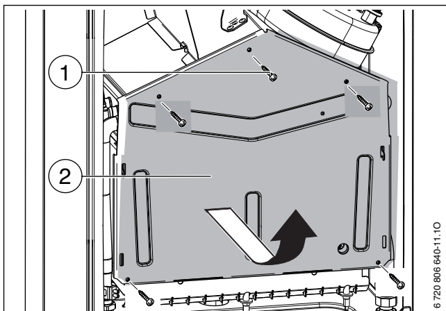
Рис. 37 Открытие горелки
