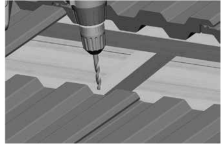
Шаг 2. Сверление отверстия в стропиле
