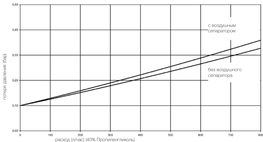
Диаграмма потери давления
