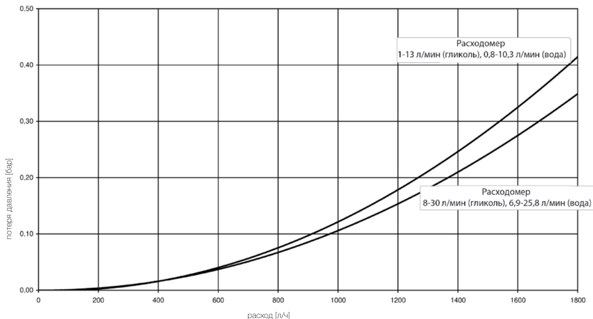
Диаграмма потери давления
