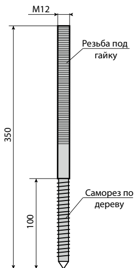
Универсальный анкер
