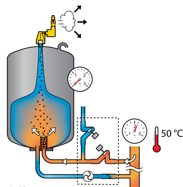
2. Нагрев системы Объем воды в системе и давление повышаются. Устройство открывает электромагнитный клапан. Вода подается в бак без давления. В баке происходит процесс деаэрации воды (падение давления и прохождение через Pall-кольца)
