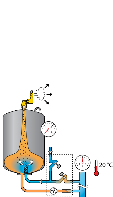
1. Начало работы Небольшой объем воды в автомате. Устройство в состоянии покоя.
