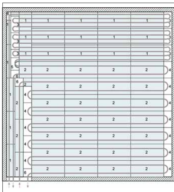
Рис. 3-59 Пример укладки при «сухом» способе монтажа
