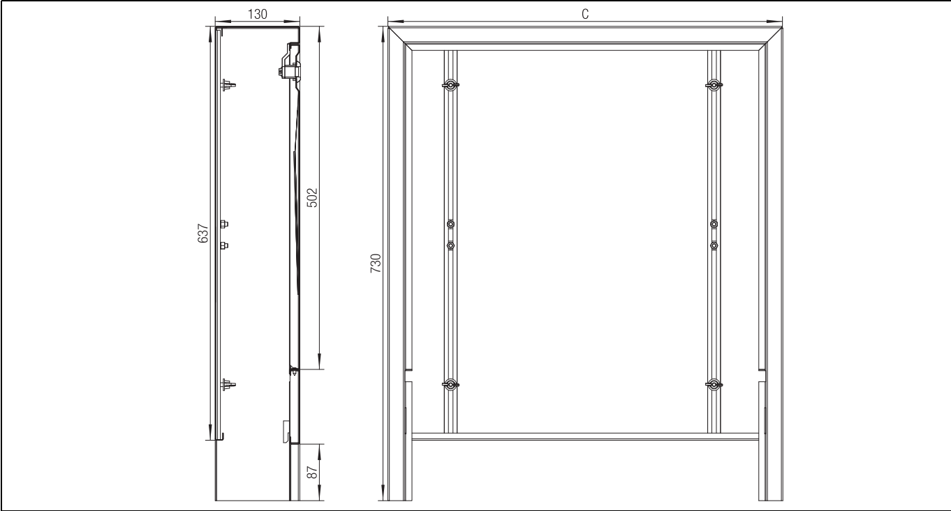
Рис. 9-13 Размеры распределительного шкафа AP C Ширина корпуса изнутри
