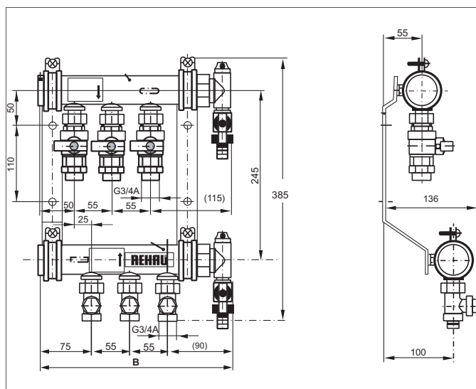
Рис. 17-2 Размеры распределительного коллектора
