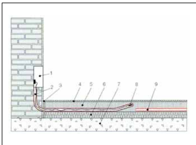
Рис. 10-34 Установка датчика температуры пола FT-НС
