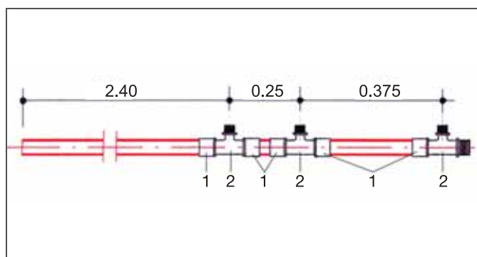
Рис. 14-11 Трубный распределитель REHAU
