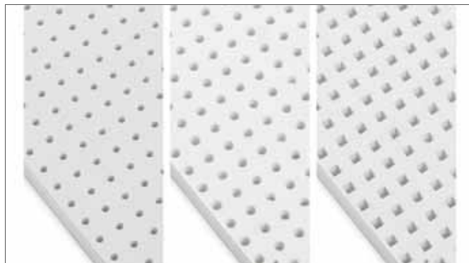
Рис. 4-2 Образцы отверстий (слева направо: 6/18 R; 8/18 R; 8/18 Q)
