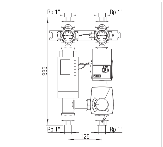
Рис. 10-8 Размеры станции температурного регулирования TRS-20
