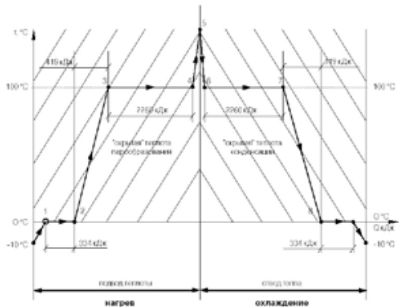
Рис. 1: График фазового перехода воды.
