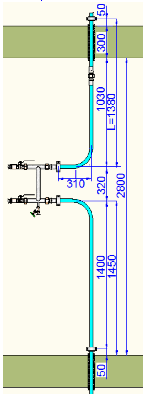
Рис.4.2.4.р.13 Этаже-стояк ГВС
