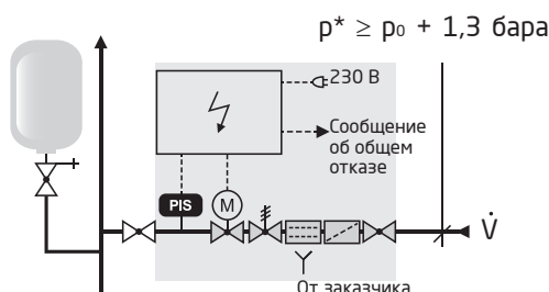
Схема Fillcontrol Plus Compact
