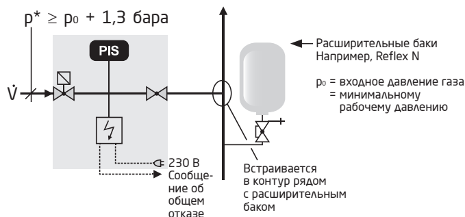
Схема Fillcontrol Plus Compact
