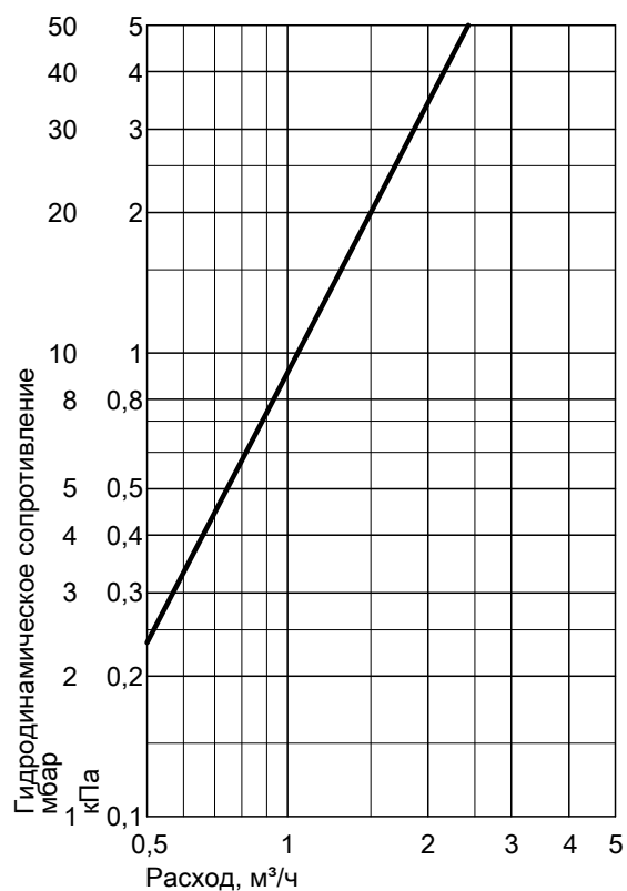
Гидродинамическое сопротивление греющего контура
