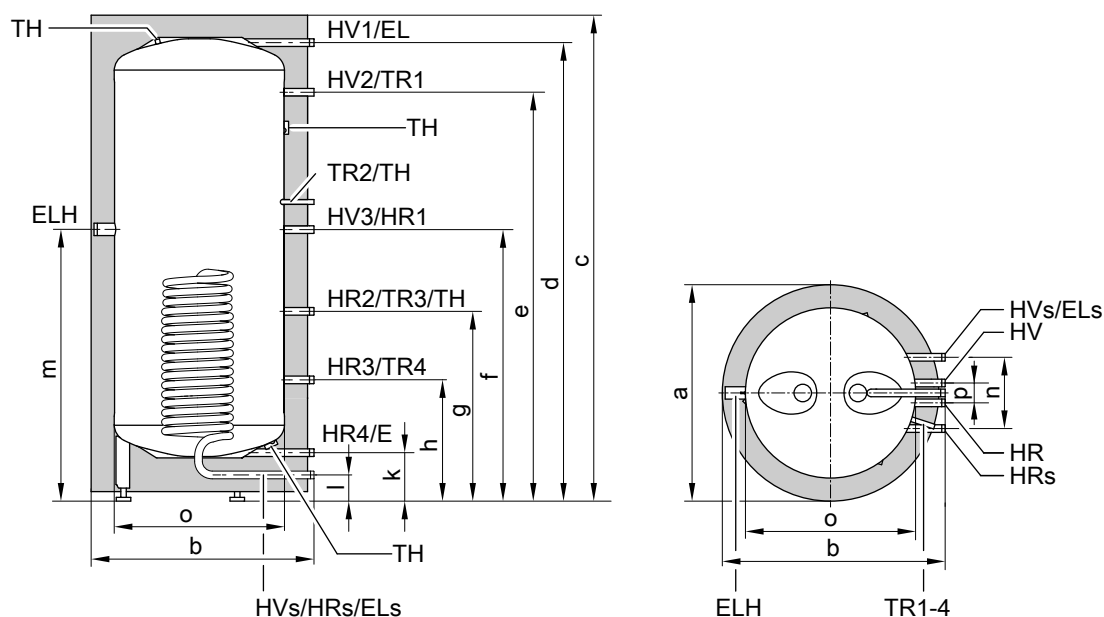
Vitocell 140-E (тип SEIA, 750 и 950 литров)
