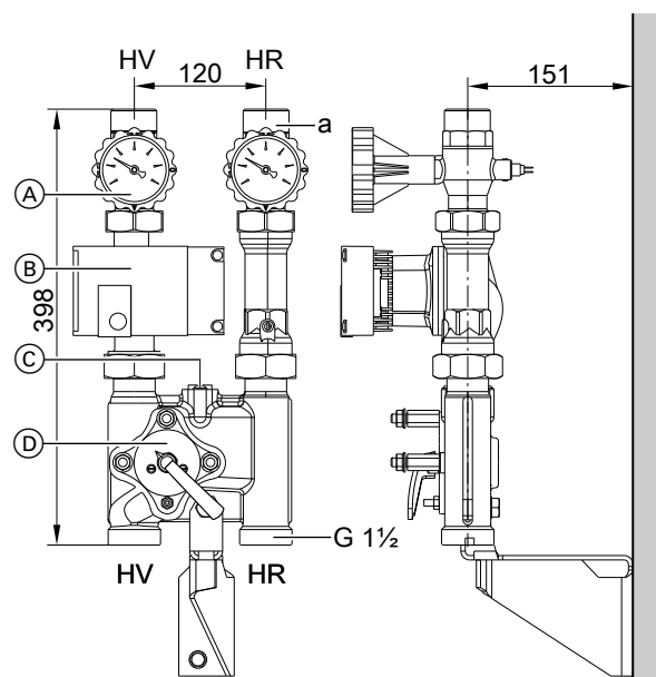
Divicon со смесителем (настенный монтаж, изображен без теплоизоляции и без комплекта привода смесителя)
