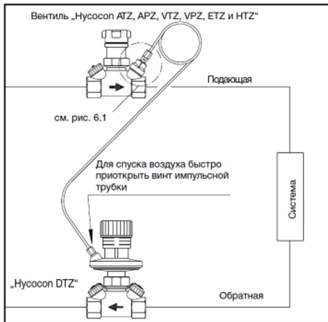
Рис. 6.2: „Нусосоп DTZ“, установка на обратной линии
