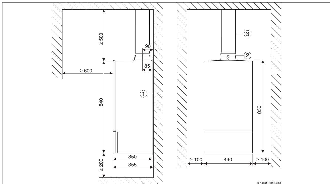
Рис. 7 \varnothing 80/125 мм, плоская крыша
