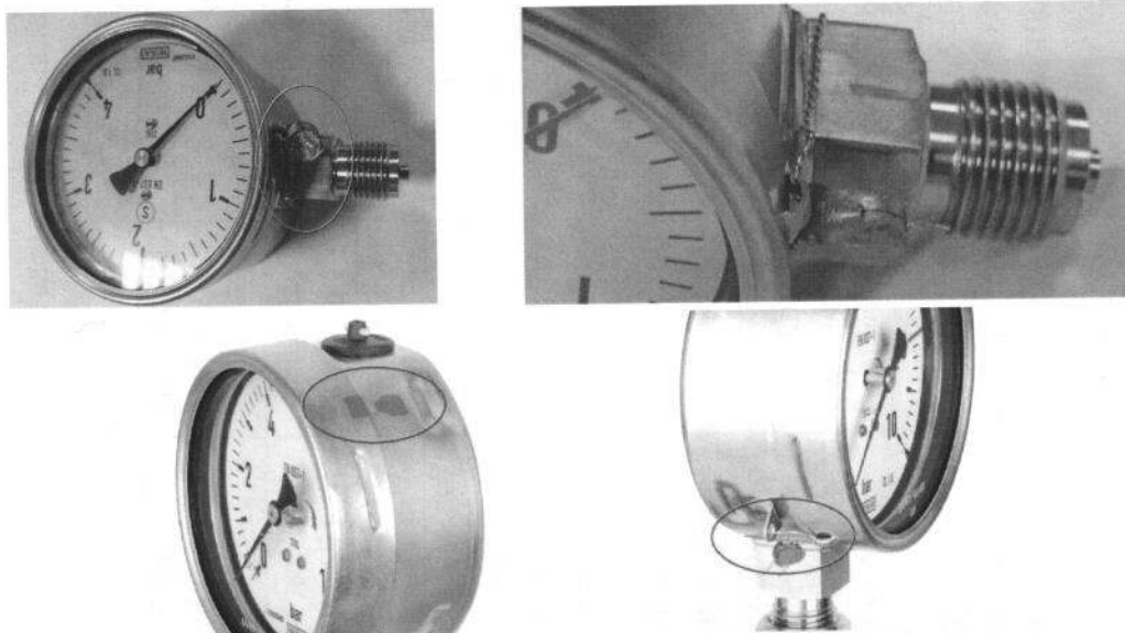
Рисунок 2 - Варианты пломбирования
