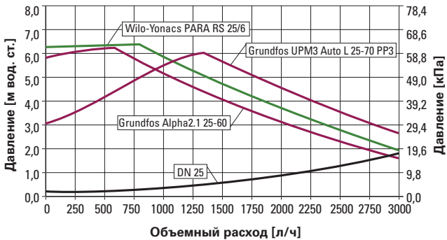
Насосная группа без смешения К31 DN25
