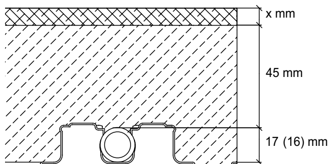
панель с бобышками x-net economic. Система в разрезе
