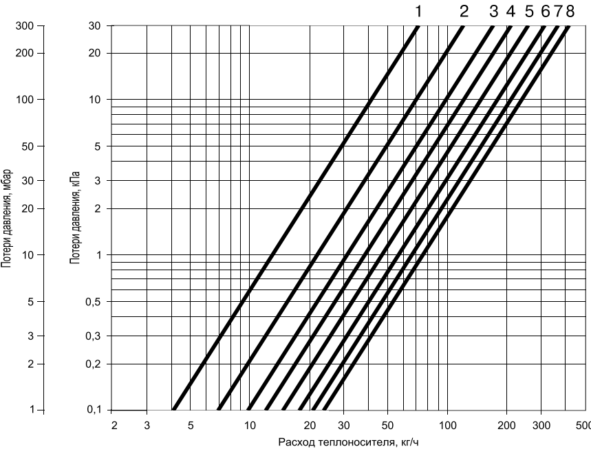
Диаграммы для термостатического клапана без узла нижнего подключения при 2 °C
