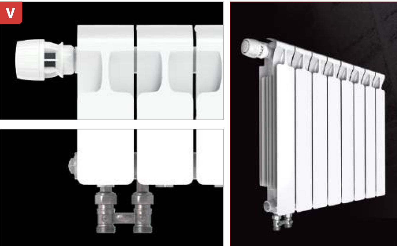
РАДИАТОРЫ ДЛЯ НИЖНЕГО ПОДКЛЮЧЕНИЯ RIFAR VENTIL на фото представлено исполнение VENTIL для радиатора MONOLIT 500
