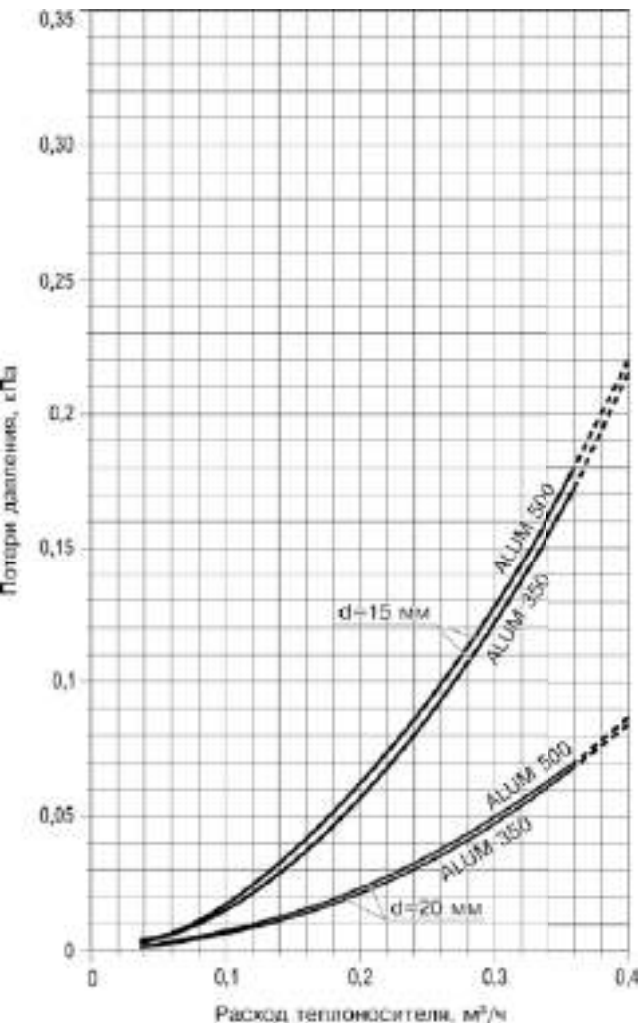
ГРАФИК ПОТЕРЬ ДАВЛЕНИЯ ΔP, кПа ОТ РАСХОДА ТЕПЛОНОСИТЕЛЯ M, м³/ч
