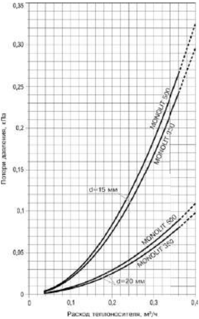
ГРАФИК ПОТЕРЬ ДАВЛЕНИЯ ΔР, кПа ОТ РАСХОДА ТЕПЛОНОСИТЕЛЯ М, м³/ч
