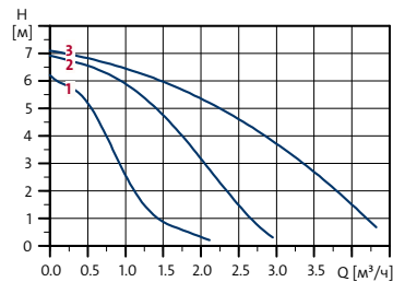
UPS 25-70/UPS 32-70 180
