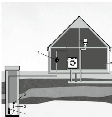
Пример монтажа насосов SB с блоками автоматики PM 1/PM 2 в колодце
