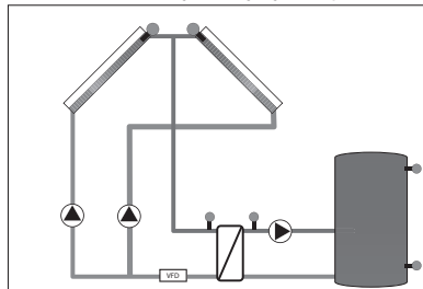
Подключение аккумулятора тепла с простым принципом накопления к двум коллекторным полям
