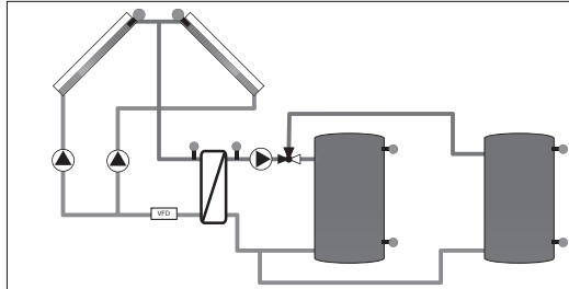
Подключение двух аккумуляторов тепла при раздельном накоплении к двум коллекторным полям
