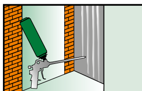
Фиксация панелей
