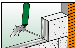
Возведение стен
