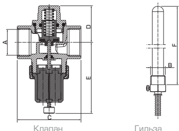
Клапан
