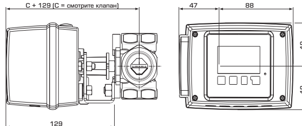
Установочные размеры для контроллера серии 90С со смесительными клапанами ESBE серий MG, G, F, T/TM, H/HG и BV
