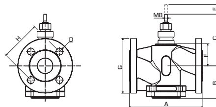
VLC225 2-ходовой со штекером компенсации давления
