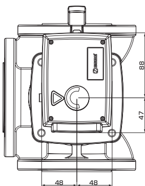
Установочные размеры для приводов серии CRA120 со смесительными клапанами ESBE серий MG, G, F, T/TM, H/HG и BIV
