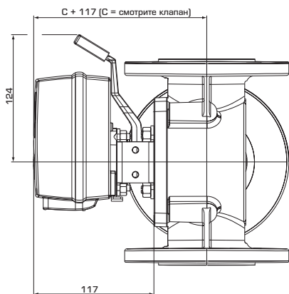
Установочные размеры для приводов серии CRC120 со смесительными клапанами ESBE серий MG, G, F, T/TM, H/HG и BIV
