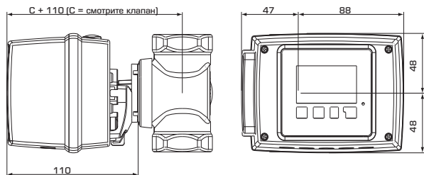
Установочные размеры для контроллера серии 90С со смесительными клапанами ESBE VRG100, VRG200, VRG300, VRH100 и VRB100
