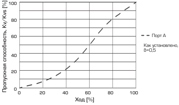
2-ходовые клапаны, DN65-150
