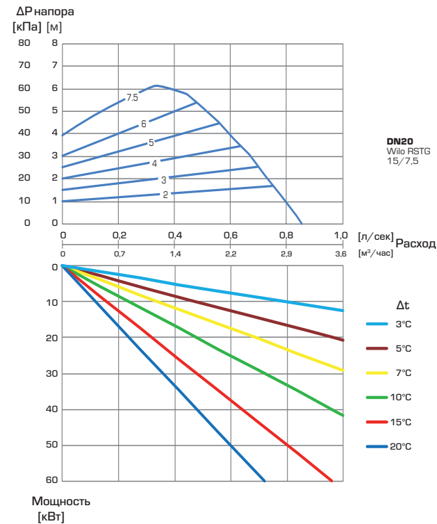
Диаграмма встроенного насоса
