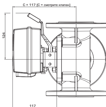
Установочные размеры для приводов серии CRA120 со смесительными клапанами ESBE серий MG, G, F, T/TM, H/HG и BIV
