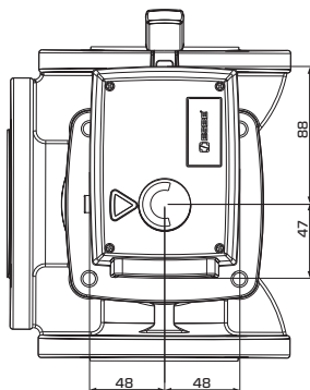
Установочные размеры для приводов серии CRC120 со смесительными клапанами ESBE серий MG, G, F, T/TM, H/HG и BIV
