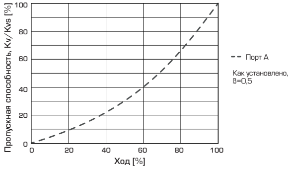
2-ходовые клапаны, DN15-50
