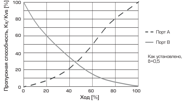
3-ходовые клапаны, DN65-150
