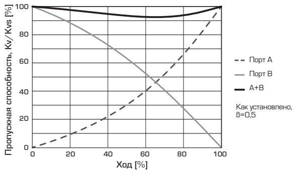
3-ходовые клапаны, DN15-50
