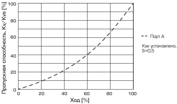
2-ходовые клапаны, DN15-50
