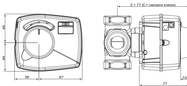
Установочные размеры для контроллеров серии CRA140 со смесительными клапанами ESBE VRG100, VRG200, VRG300, VRH100 и VRB100
