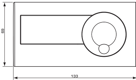
Установочные размеры для комнатного модуля
