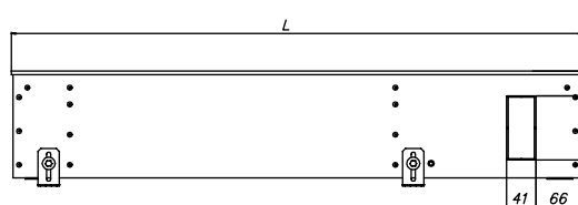
ЕКN.240.200, вид сбоку
