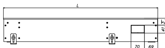
EKN.300.120, вид сбоку
