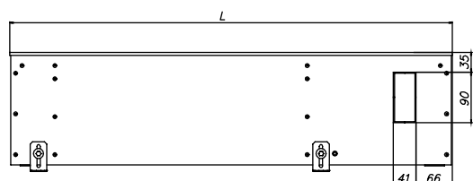
EKN.300.200, вид сбоку
