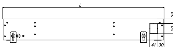
ЕКQ.190.150, вид сбоку
