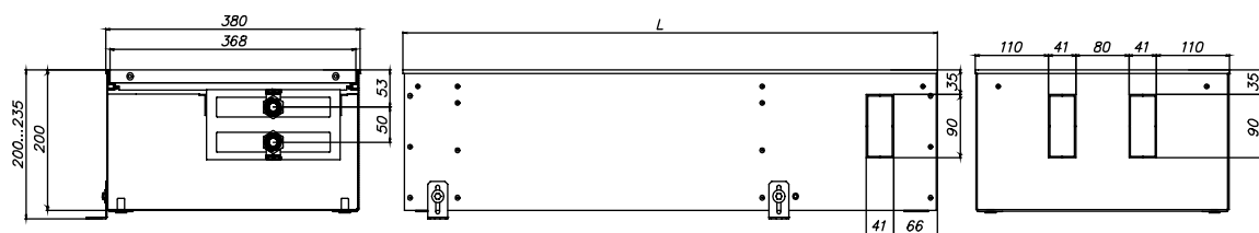
ЕКН.380.200, вид сбоку
