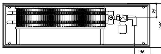
ЕКN.240.150, вид сбоку
