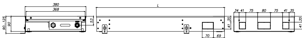
ЕКН.380.120, вид сбоку
