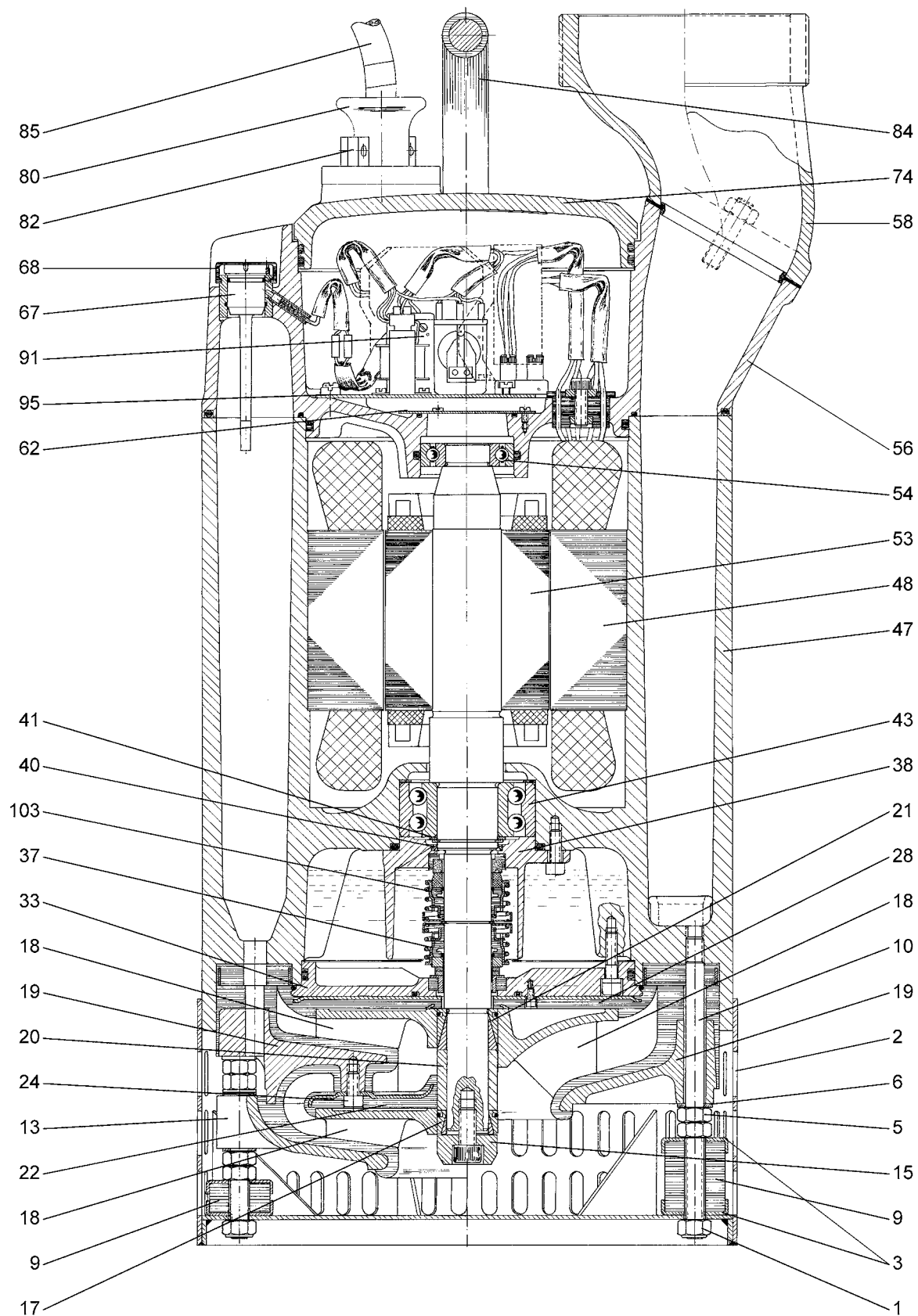
Рис. 136. DW.100.110.(A)3.H/150.110.(A)3
