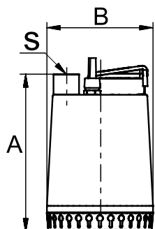
Рис. 16. Габаритные размеры
