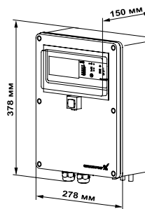
Рис. 123. Габаритные размеры
