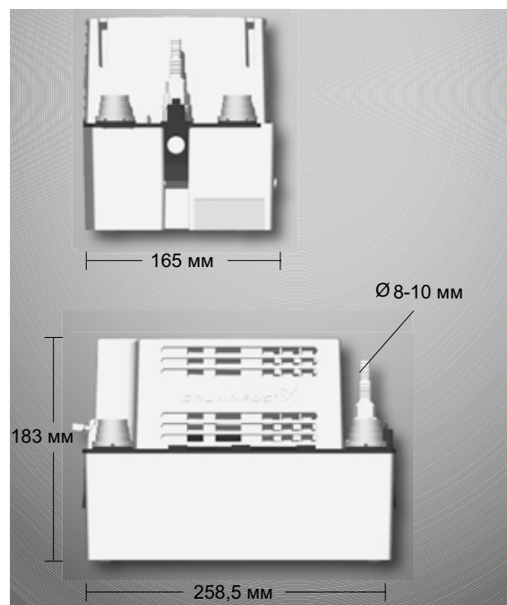
Рис. 76. Габаритные размеры
