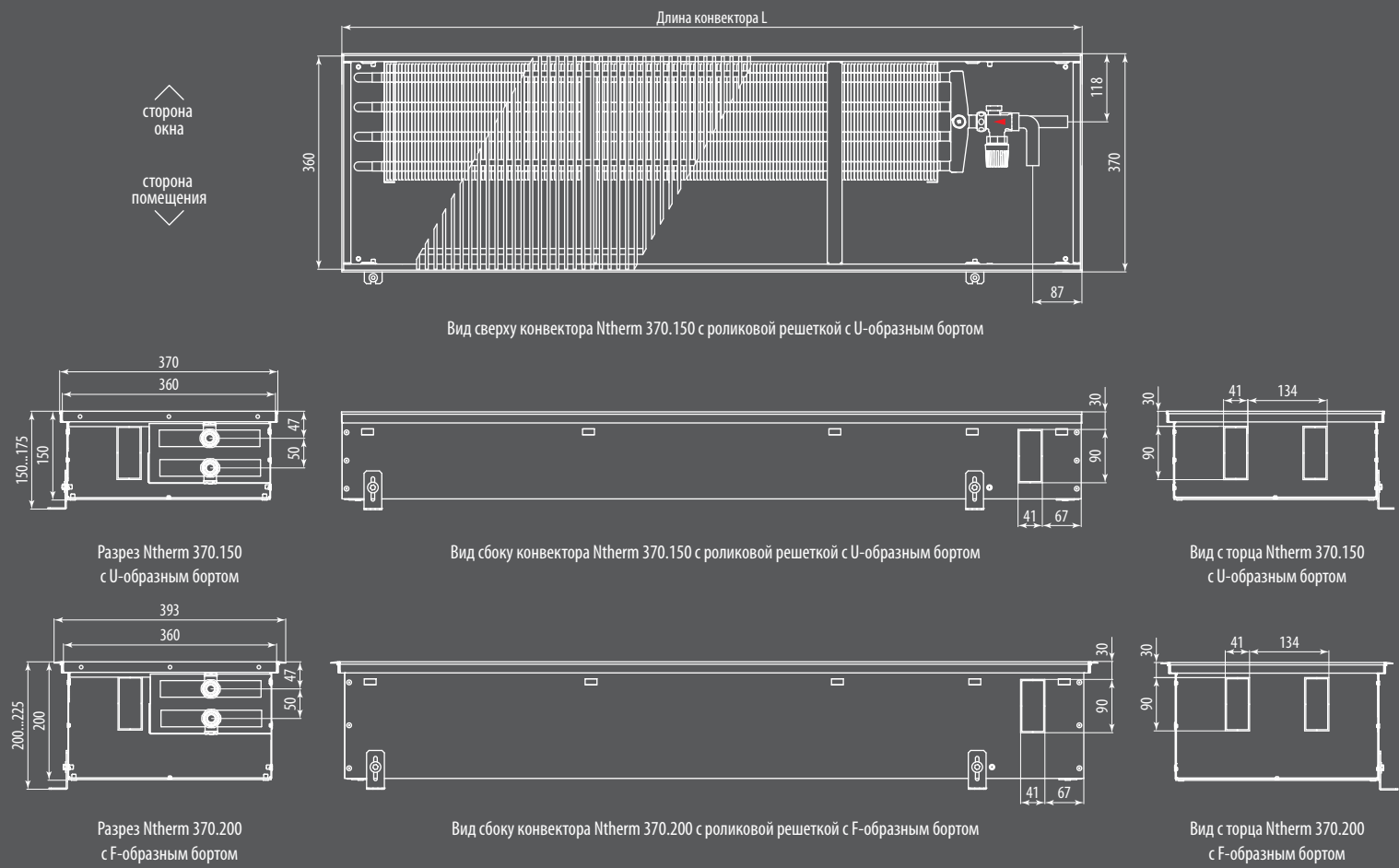
Размеры Ntherm 370.150 и Ntherm 370.200
