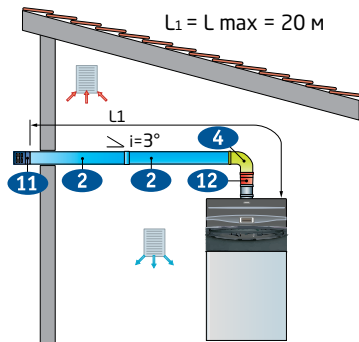
Вывод дымовой трубы через стену
