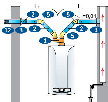
С забором воздуха с улицы
