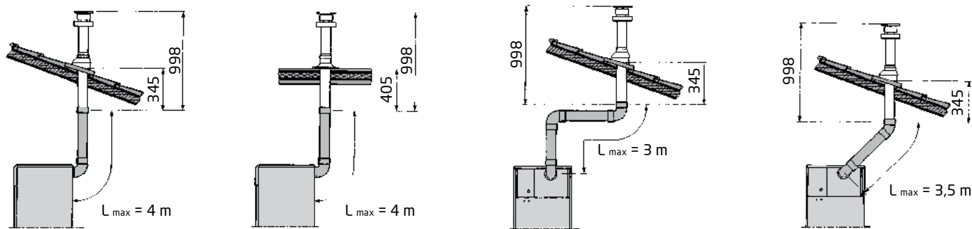
Коаксиальная труба с вертикальным выходом
