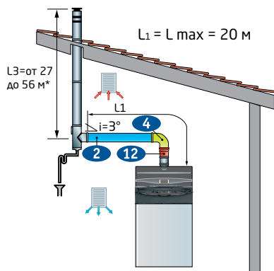
Вывод дымовой трубы в дымоход
