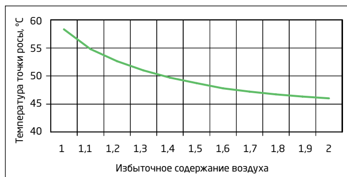
Рис. 2. Зависимость точки росы от избыточного содержания воздуха при использовании в качестве топлива природного газа (метана).
