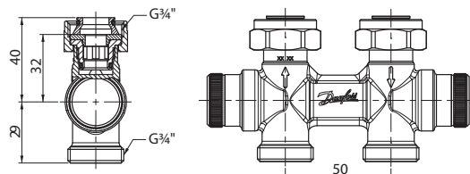
RLV-KDV угловой левый с присоединением к отопительному прибору G\frac{3}{4} "
