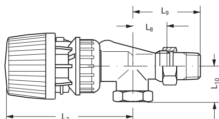
Угловой горизонтальный клапан (УК) с термостатическим элементом RTR 7090
