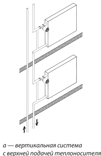
Одноконтурная насосная система отопления
