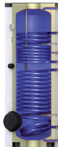
Водоподогреватель для систем с солнечным коллектором Reflex SF/2
