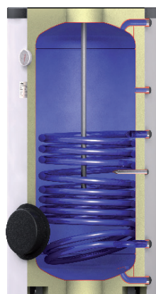
Водоподогреватель Reflex SB/SF
