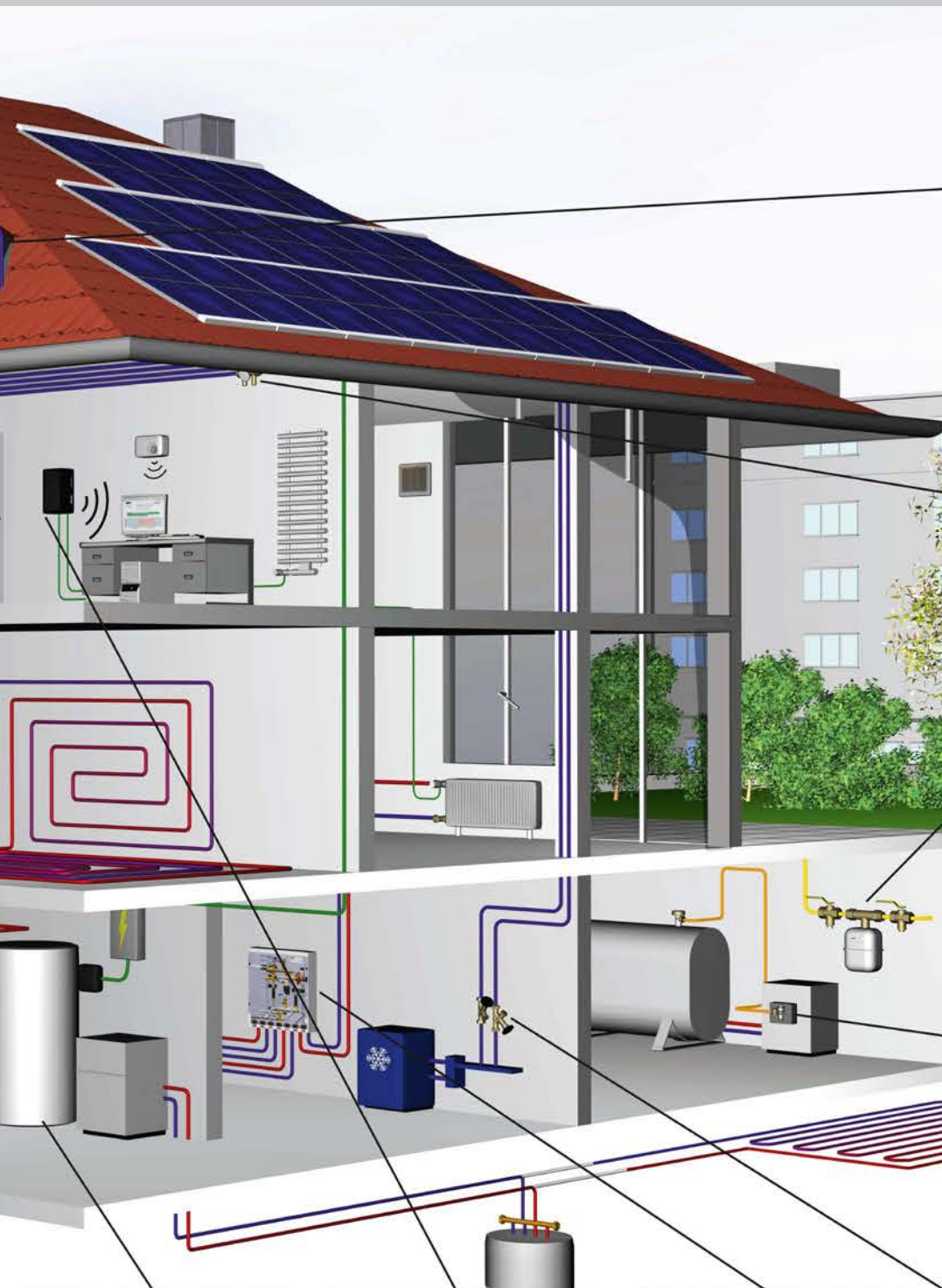
Солнечные коллекторы
