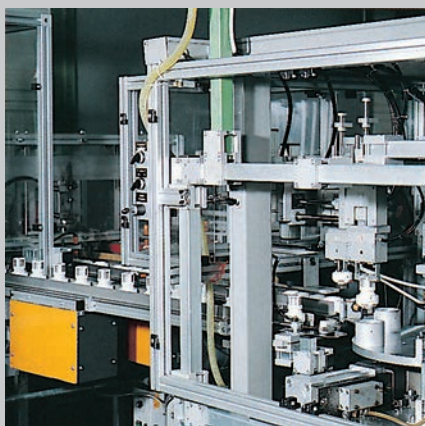
Сборочный автомат
