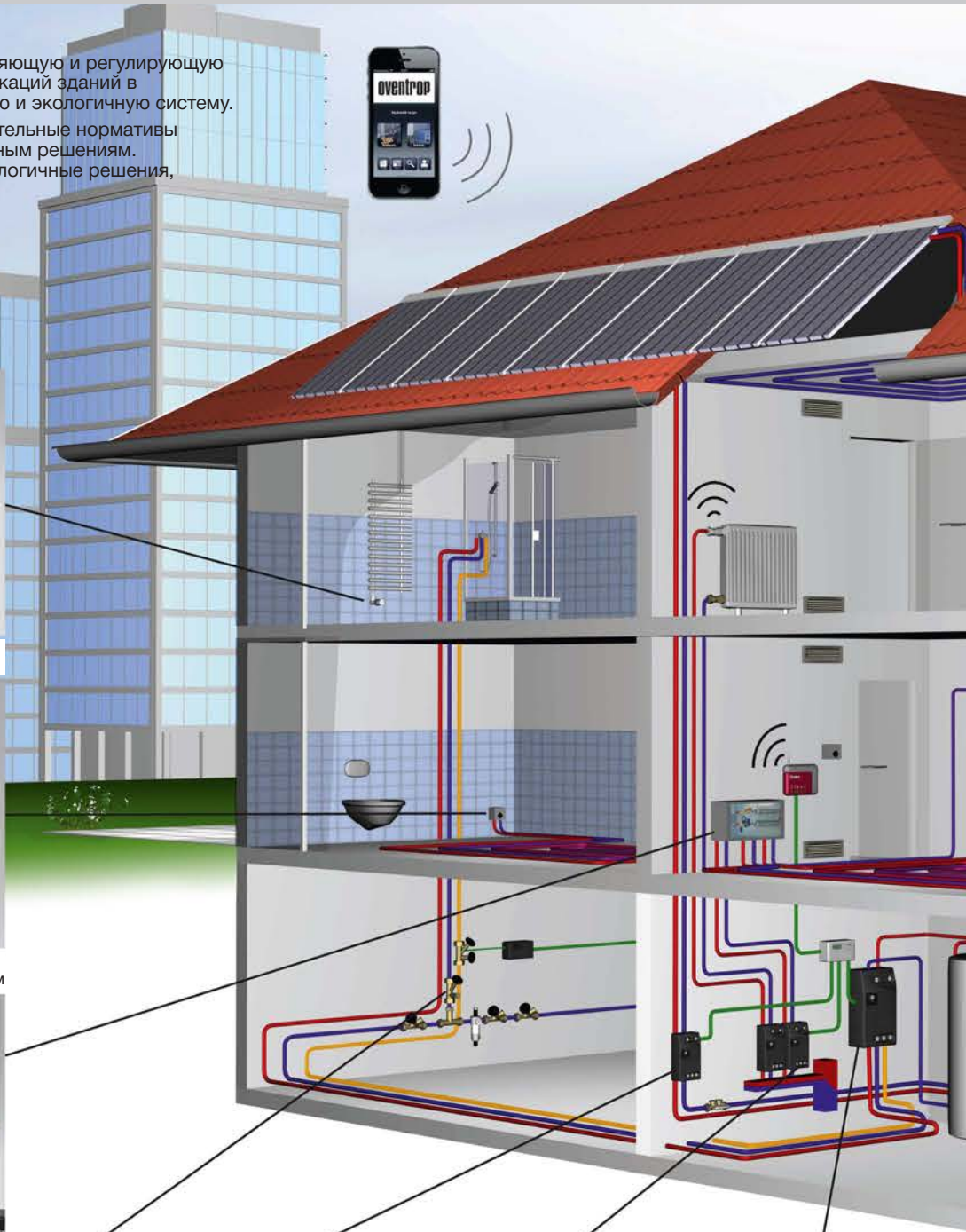
Регулирование температуры помещений с панельным отоплением
