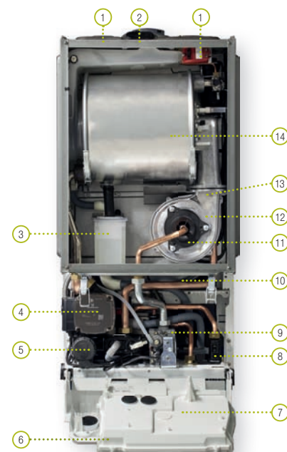
Na zdjęciu został przedstawiony model 25 C.S.I. E
