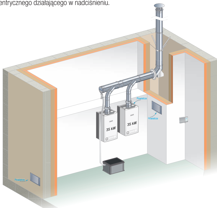
Schemat poglądowy montażu systemu spalinowego do kaskady kotłów Mynute Green 35 R.S.I. E (2 x 35 kW)
