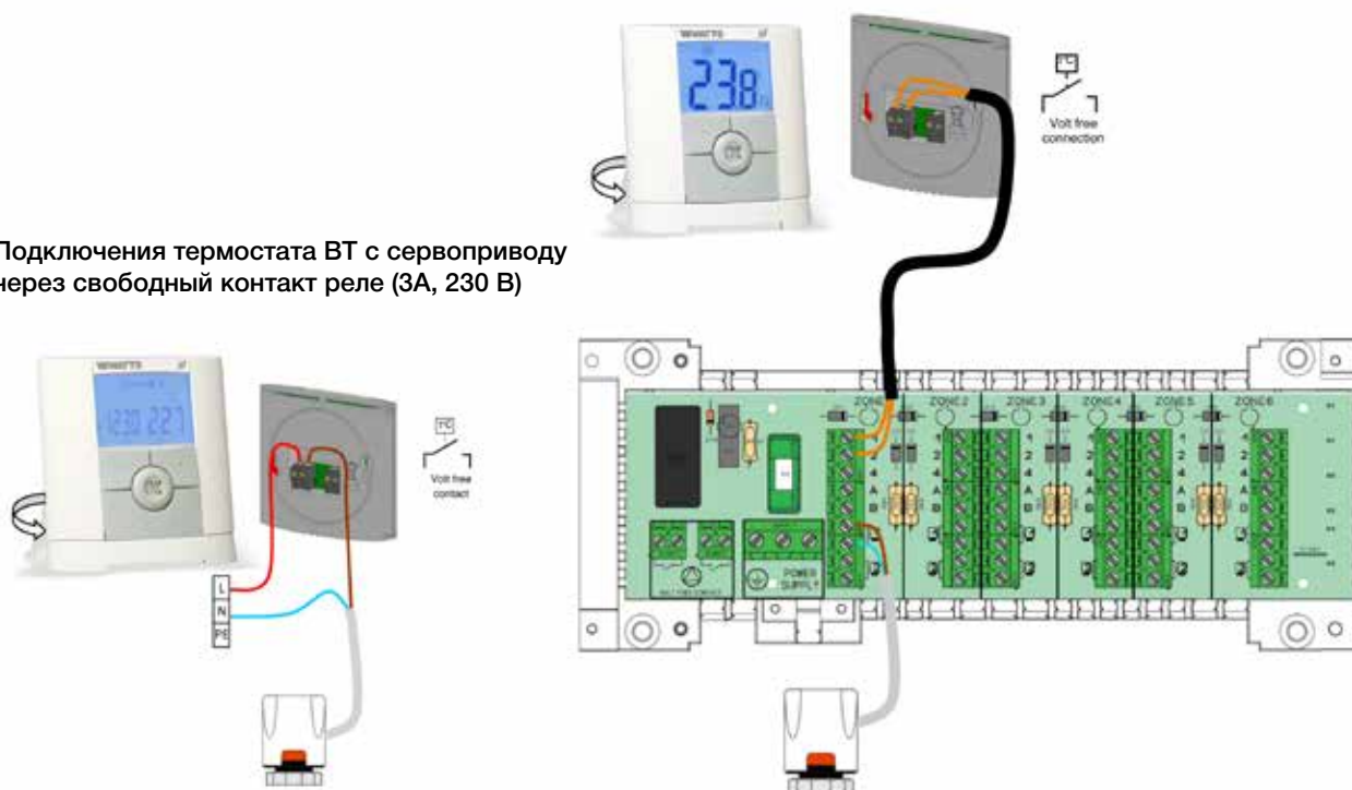
Подключение термостата ВТ к модулю WFHC через свободный контакт реле (2-жильный провод)
