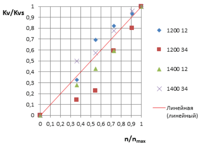
Рис. 25 - Расходная характеристика клапана
