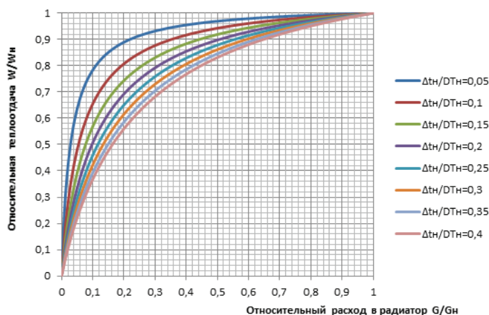
Рис. 24 - Зависимость теплоотдачи от относительного расхода
