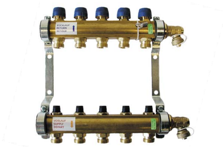
Коллектор НКV-5
