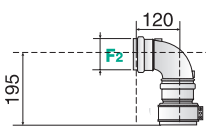
Модель FF - раздельный дымоотвод/воздуховод
