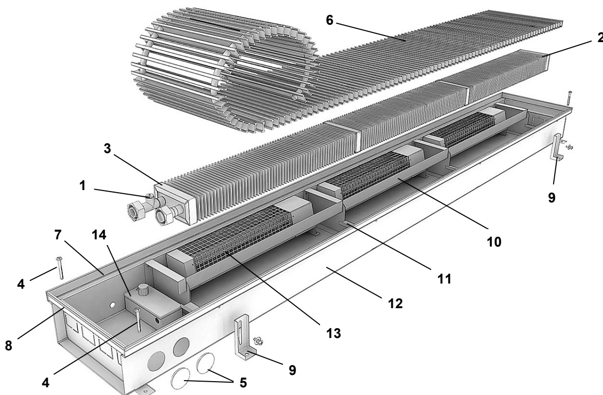
Рис. 1.4. Конструктивное устройство конвектора «VARMANN Qtherm»:
