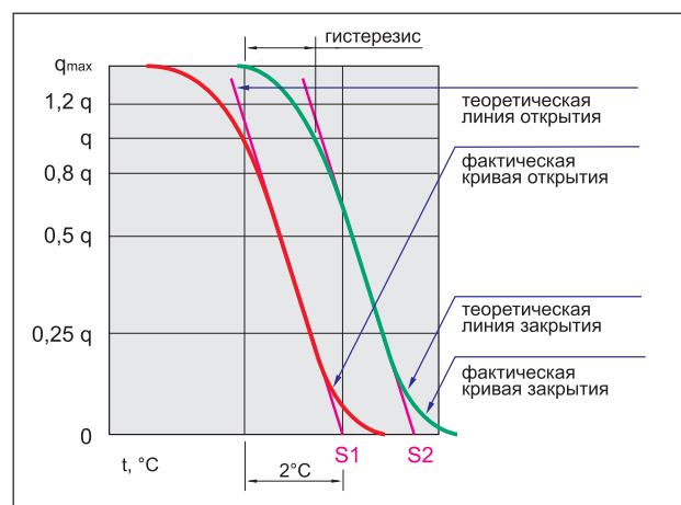
Рис.3 График закрытия и открытия термоэлемента
