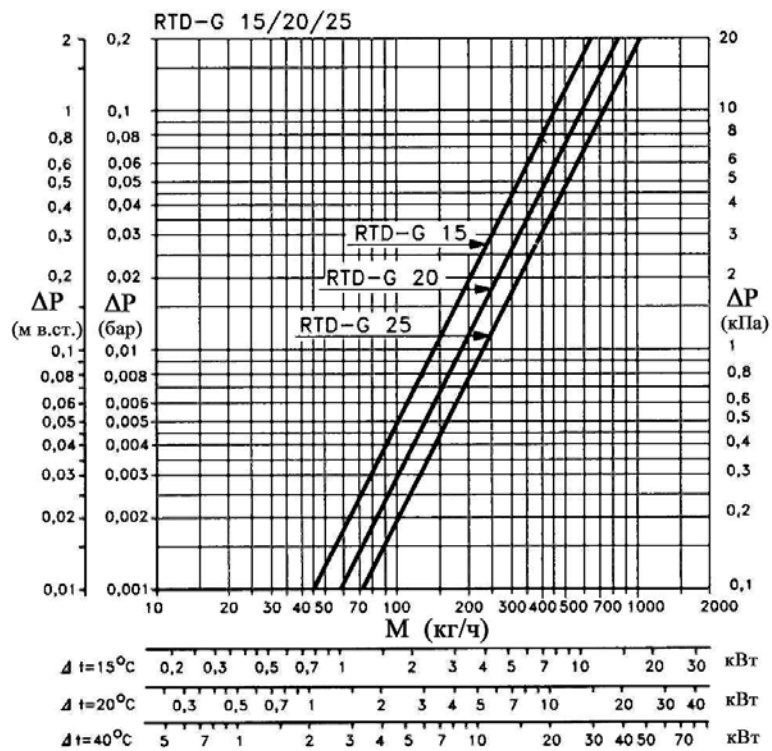
Рис. 2.2. Гидравлические характеристики термостатов фирмы «Данфосс»: а – RTD-N 15 при различных уровнях монтажной настройки клапана для двухтрубных систем отопления с подводками d_y 15 мм; б – RTD-G для гравитационных и насосных однотрубных систем отопления с подводками d_y 15, 20 и 25 мм (при настройке на режим 2К)
