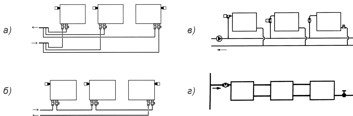
Рис. 2.3. Варианты присоединения секционных радиаторов «Zehnder Charleston» к теплопроводам при их горизонтальной разводке в системах отопления
