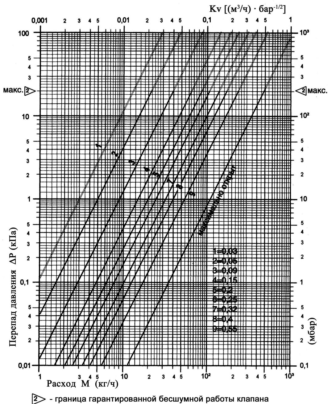
Рис. 3.1. Гидравлические характеристики термостатов «ГЕРЦ-TS-90-V» с присоединительными размерами 3/8" и 1/2" с настройкой на режим 2К (2°C) и при снятой термостатической головке (при полном открытии вентиля)
