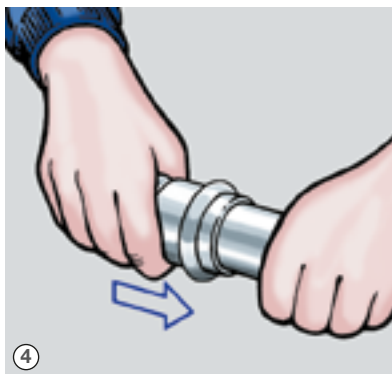
Надеть на трубу пресс-муфту до упора.
