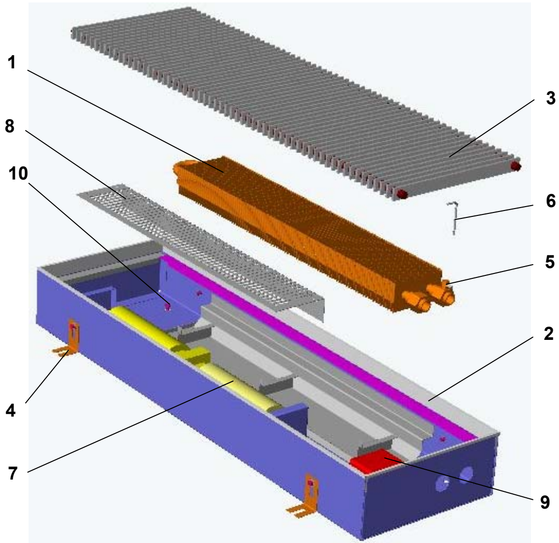
Рис. 1.1. Конвектор «Изотерм-ТД-В»:
