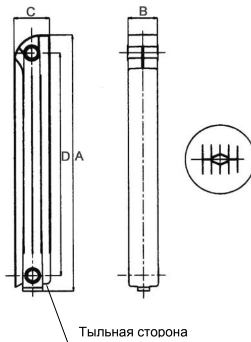
Рис. 1.4. Общий вид (a) и габаритные размеры (б) алюминиевого радиатора VOX
