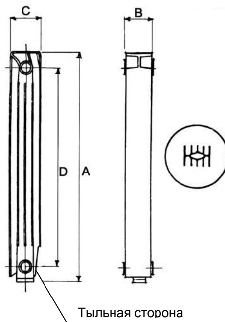
Рис. 1.1. Общий вид (а) и габаритные размеры (б) алюминиевого радиатора MIX
