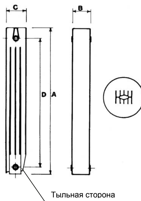
Рис. 1.2. Общий вид (а) и габаритные размеры (б) алюминиевого радиатора VIP
