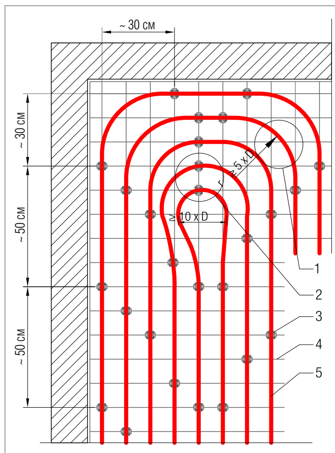
Рис. 3-46 Формирование разворотной петли в регистре отопительных труб. Пример укладки трубы RAUTHERM S 17 x 2,0 с шагом 100 мм на мат RTM 100 1 поворот на 90° 2 вершина поворота 3 поворотная клипса 4 арматурная сетка 5 труба
